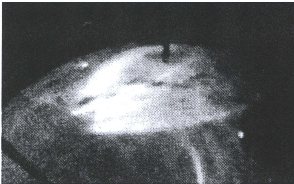
Avgaser från raket. Den 20 september 1977 fotograferades den mystiska "maneten" över Petrozavodsk av en automatisk kamera i Sodankylä i Finland. Till höger en illustration av fenomenet.
